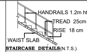
STAIRCASE DETAILS (N.T.S.)
