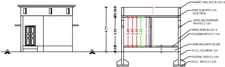
ELEVATION
