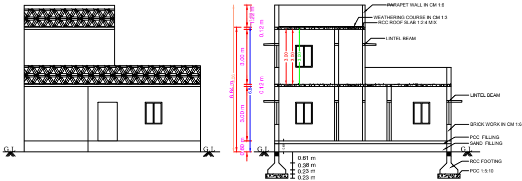
ELEVATION
