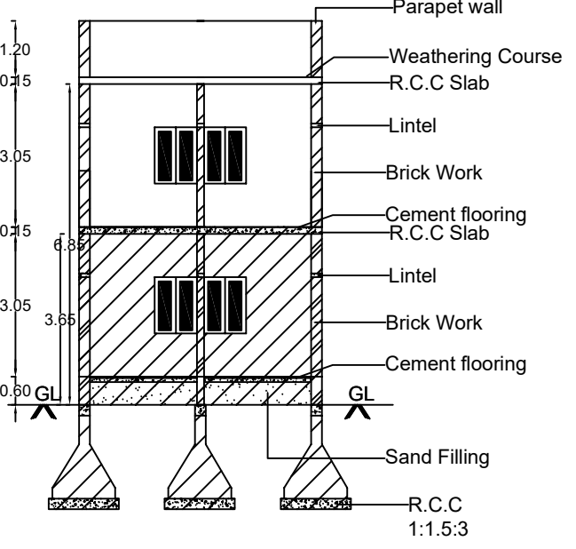
SECTION ON'AB'
