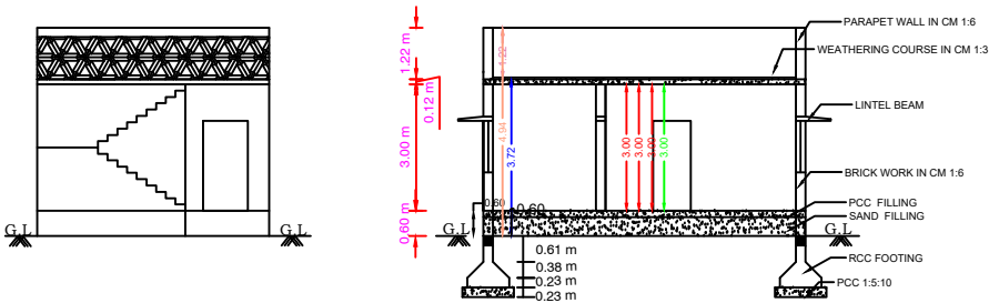
ELEVATION
