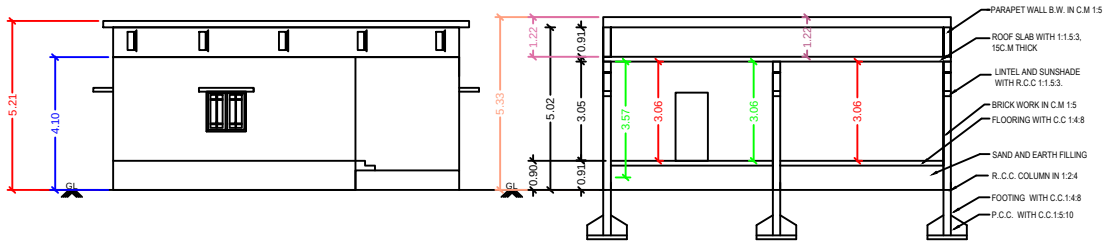
ELEVATION
