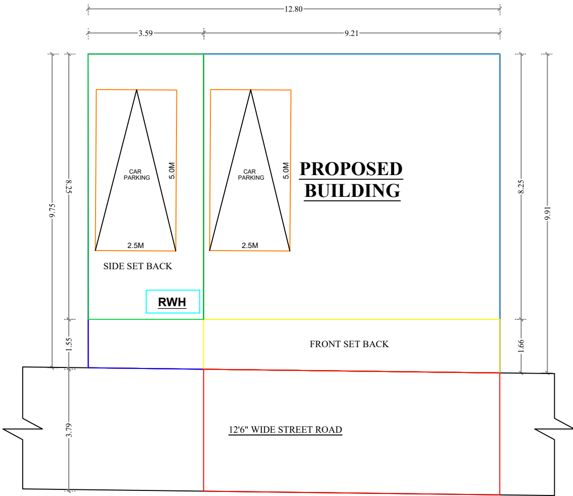
.SITE PLAN.
