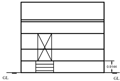
ELEVATION
