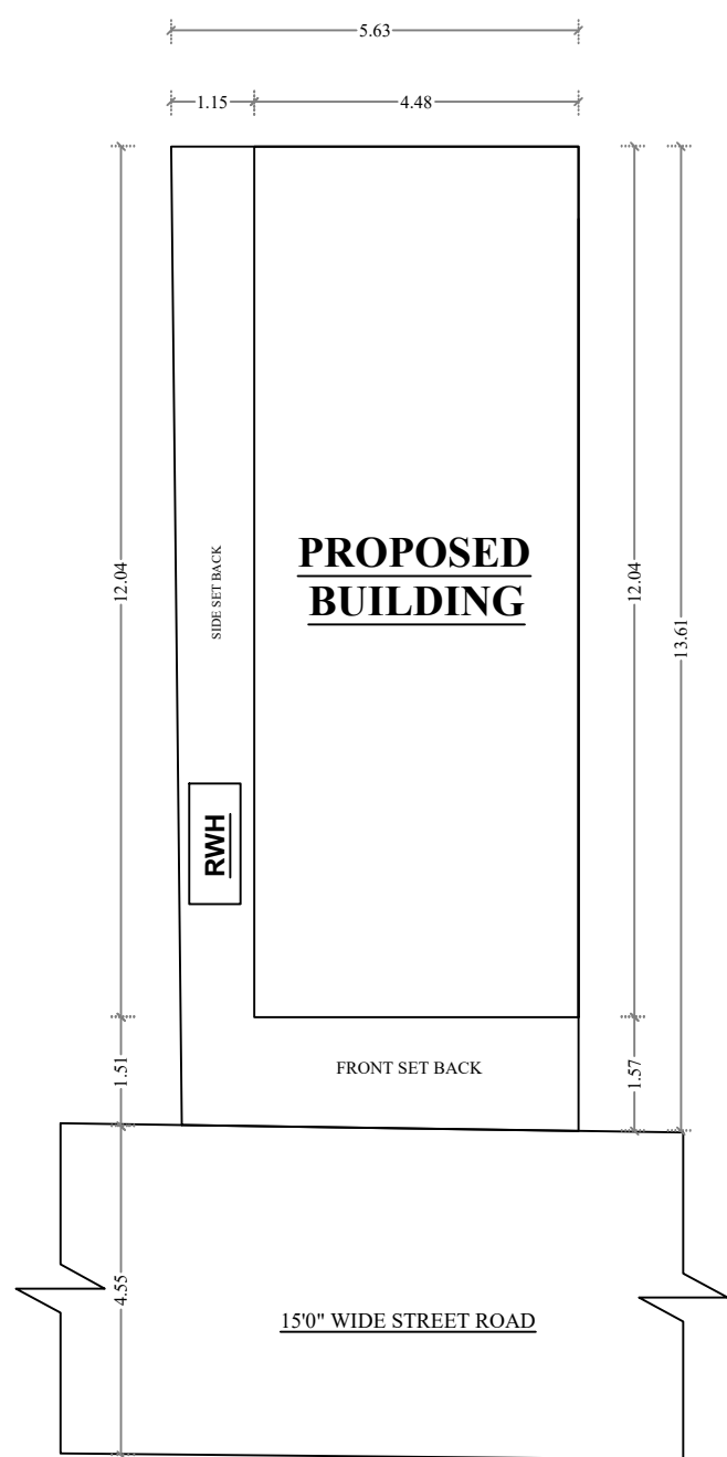
.SITE PLAN.
