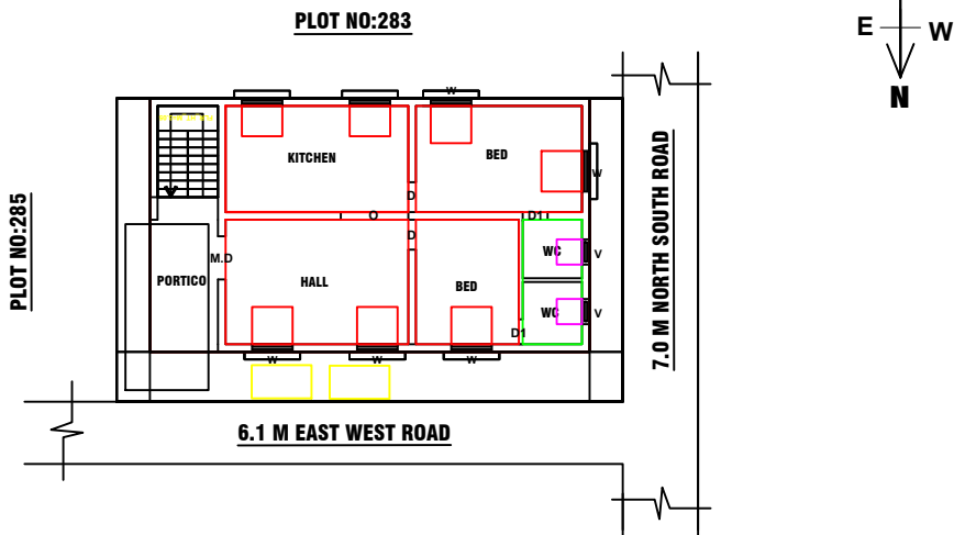
SITE PLAN:
