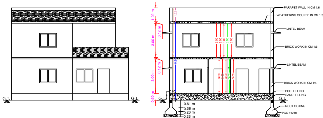
ELEVATION
