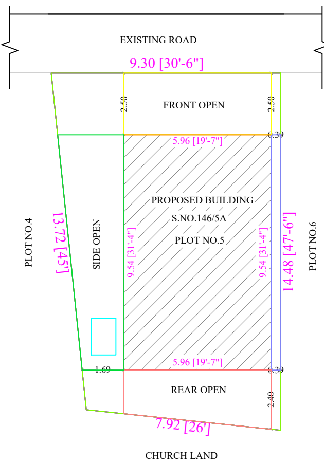
SITE PLAN :
