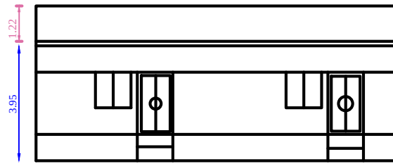
ELEVATION
