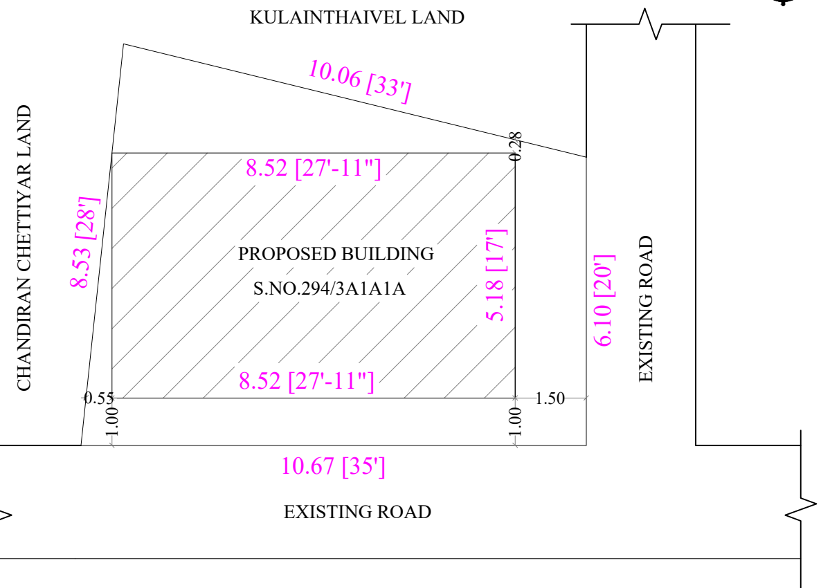
SITE PLAN :
