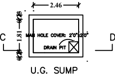
U.G. SUMP
