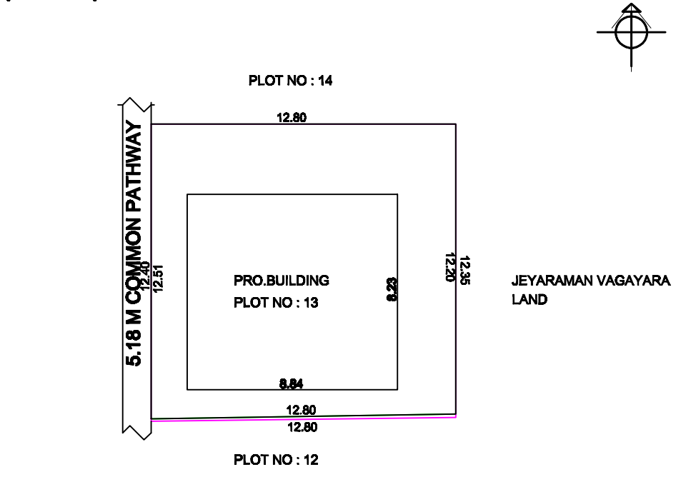
SITE PLAN :
