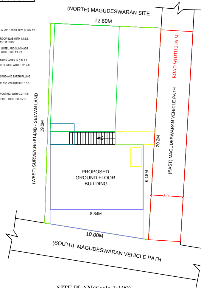
SITE PLAN(Scale 1:100)
