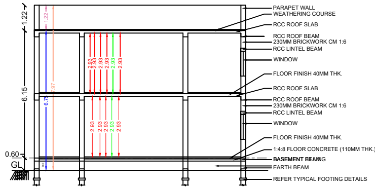
2 SECTION A-B
