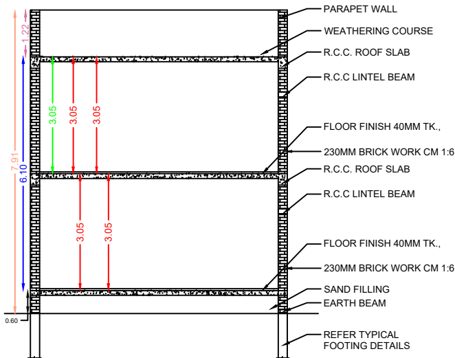
SECTION A-B
