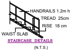
STAIRCASE DETAILS (N.T.S.)
