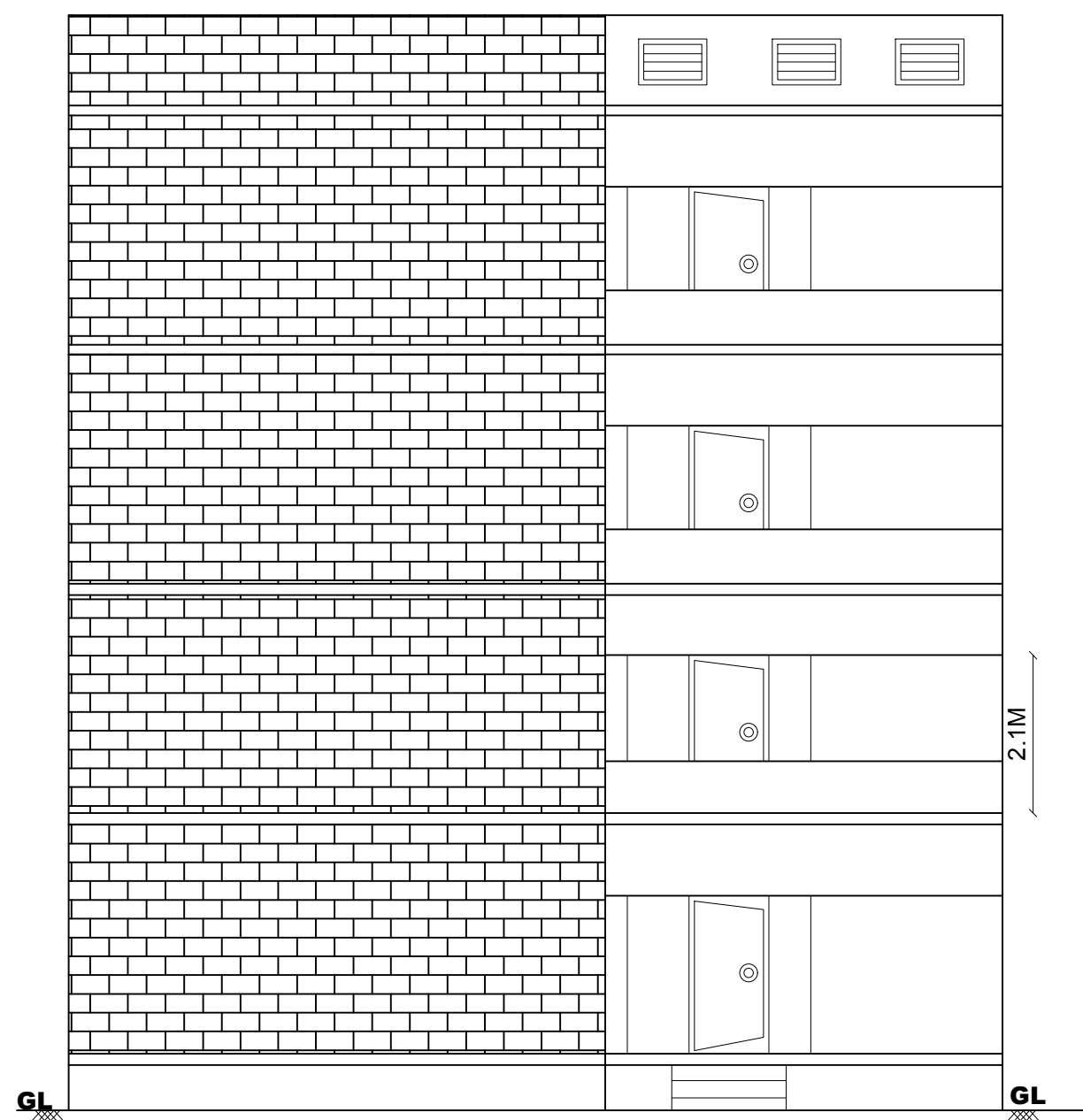
ELEVATION
