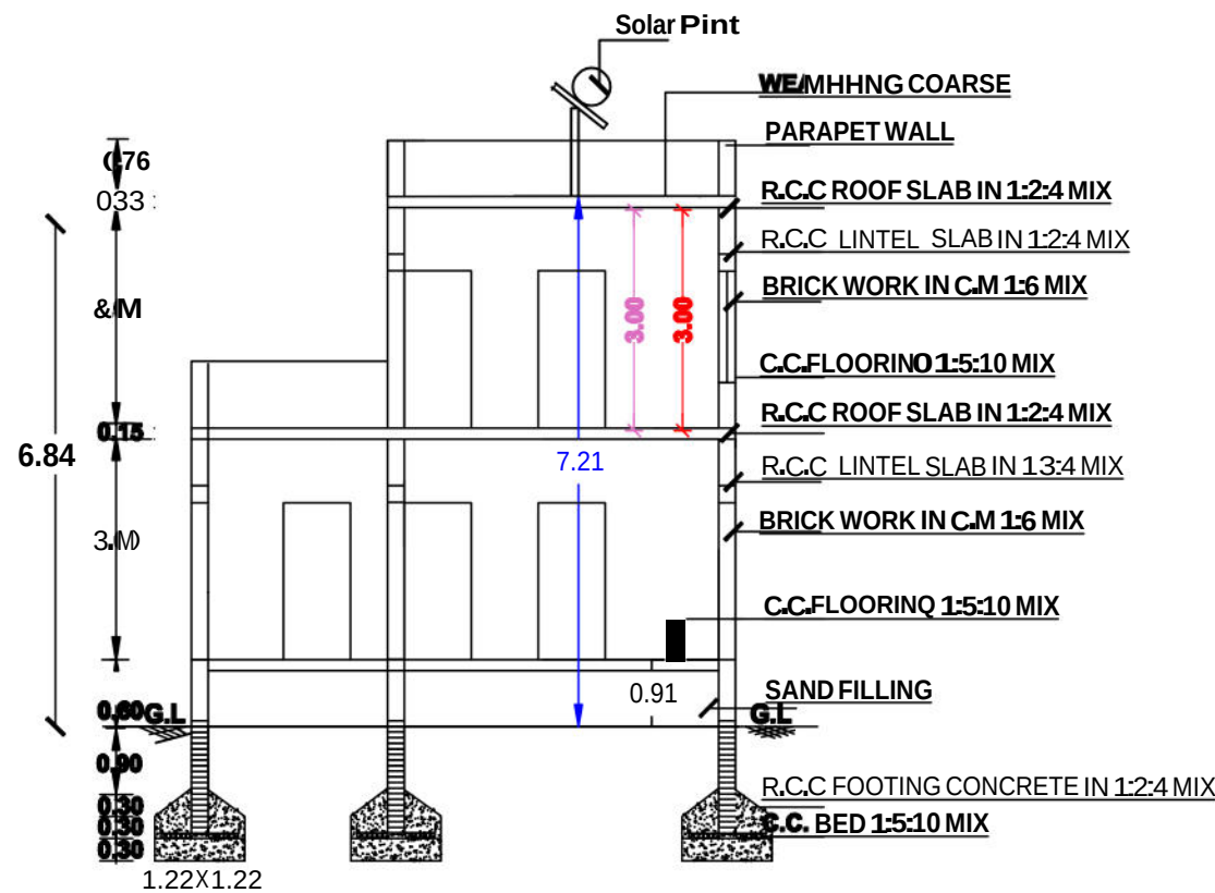
SECTION ONAB
