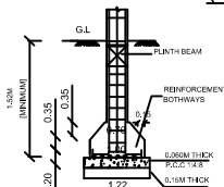
TYP. DET. COLUMN FOOTING
