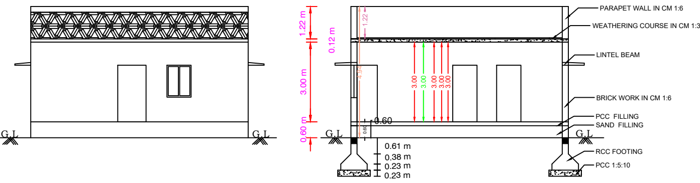
ELEVATION
