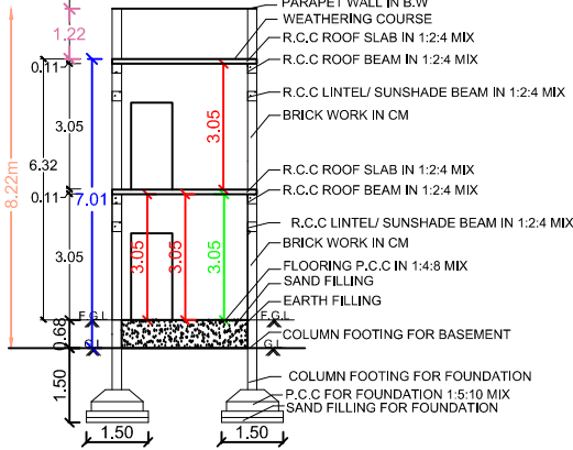
SECTION -AB
