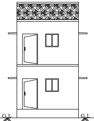
ELEVATION
