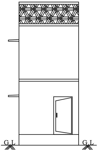
ELEVATION
