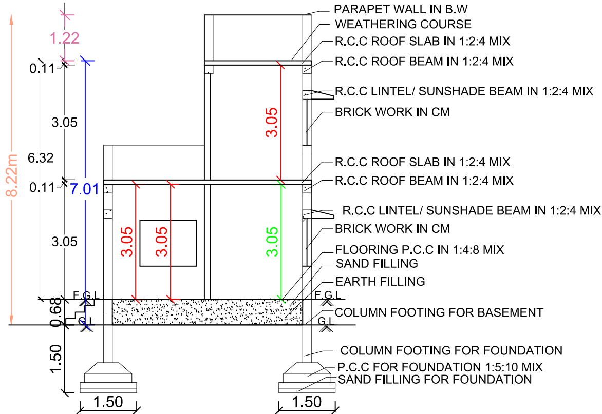
SECTION -AB
