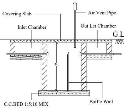
SECTION ON S.Tank [N.T.S.]
