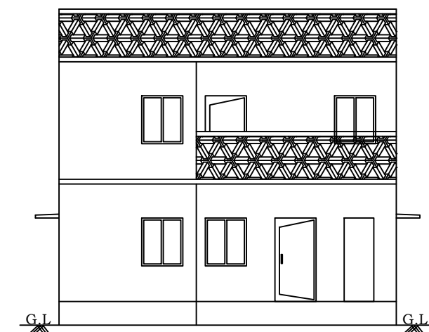
ELEVATION
