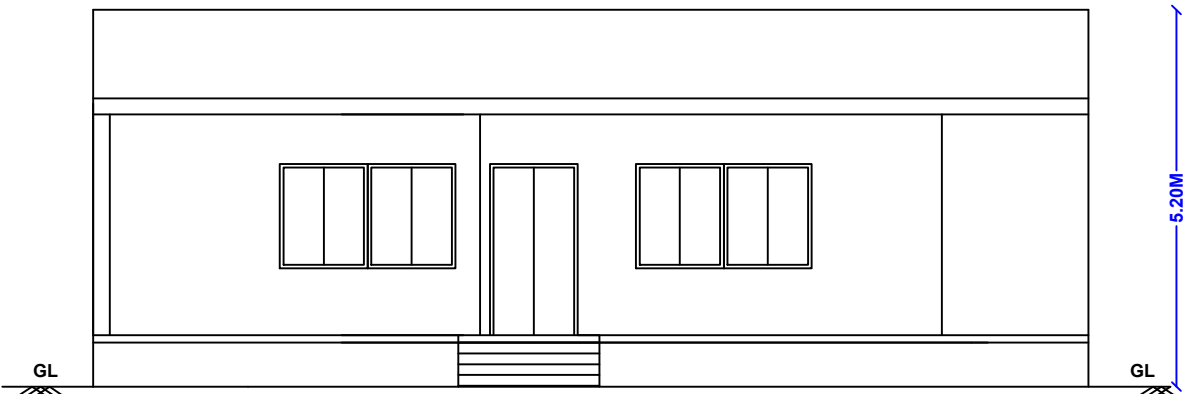
ELEVATION
