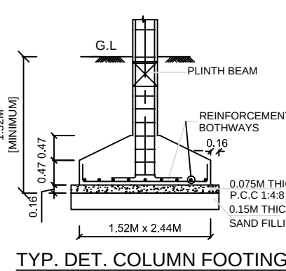
TYP. DET. COLUMN FOOTING
