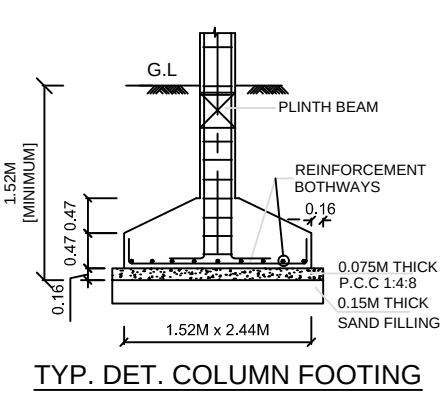
TYP. DET. COLUMN FOOTING
