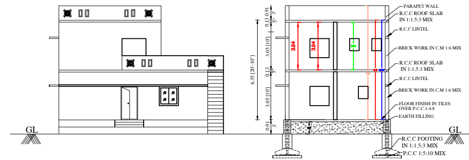
ELEVATION
