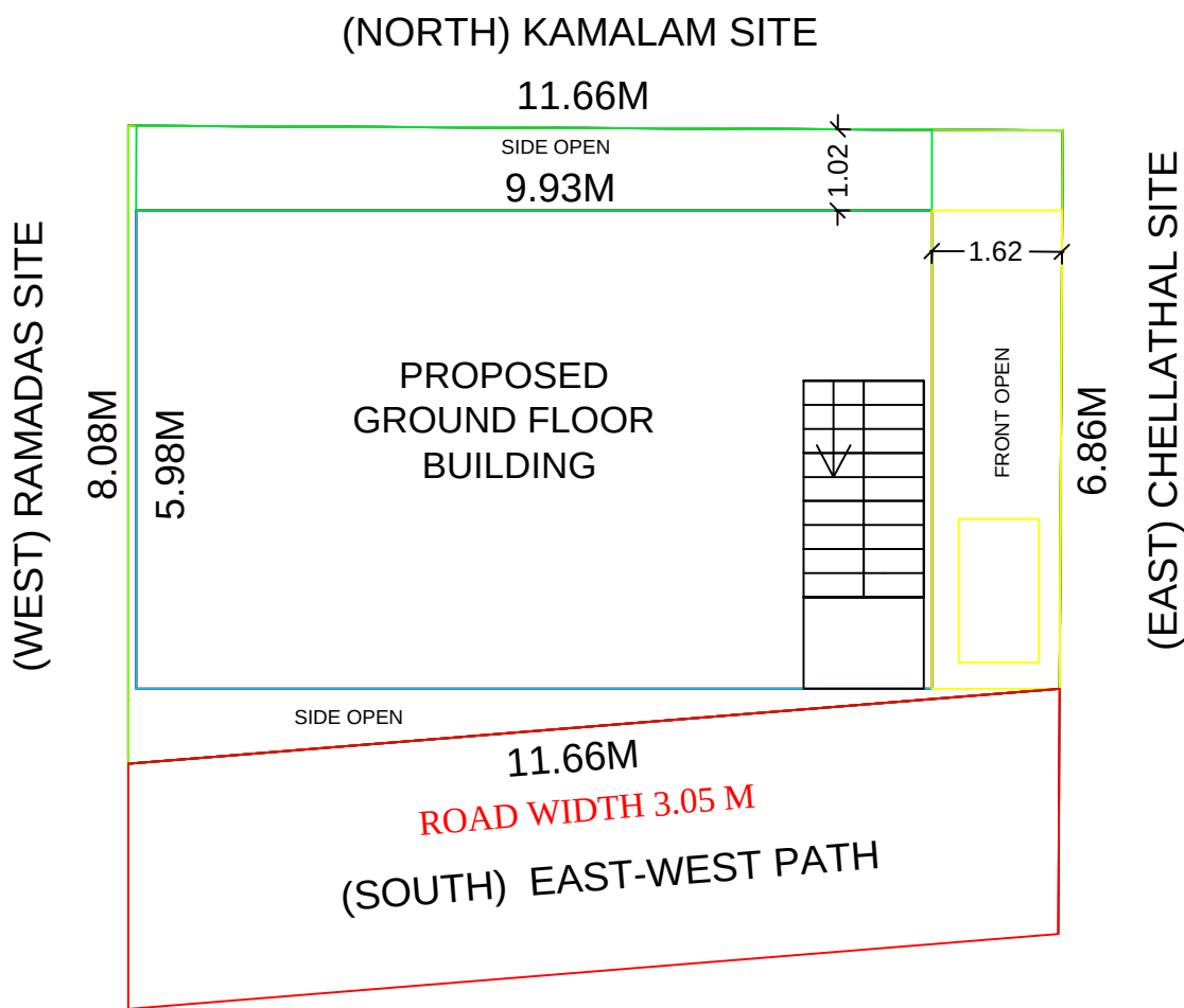
SITE PLAN(Scale 1:100)
