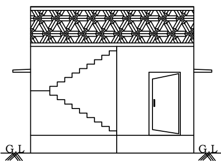
ELEVATION
