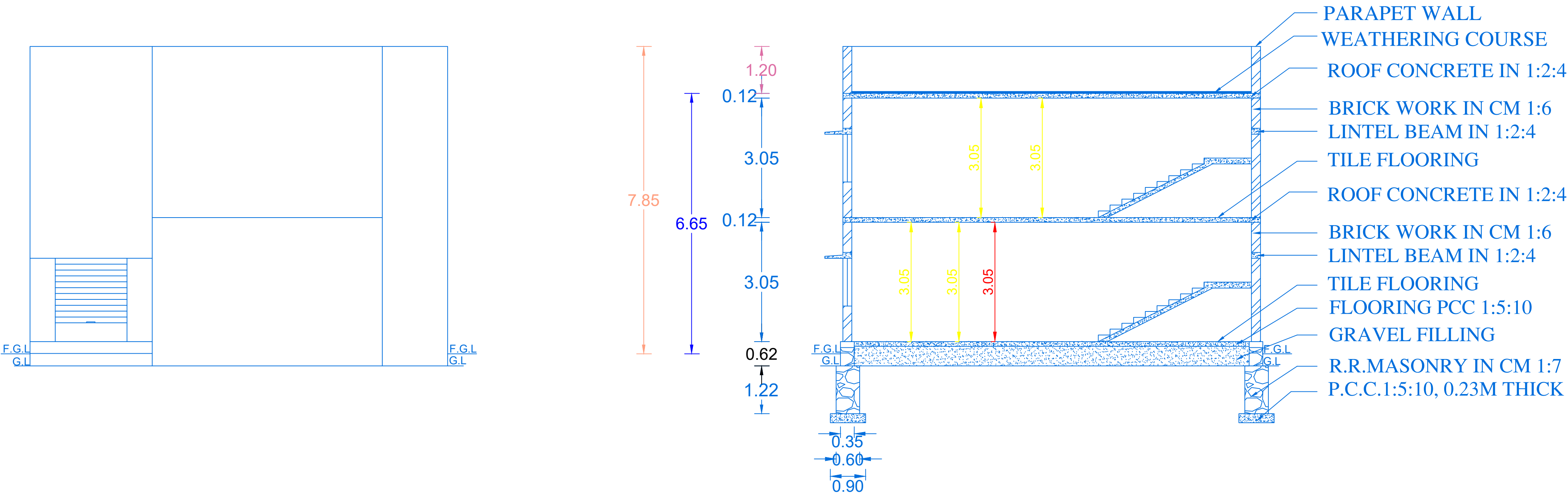
ELEVATION
