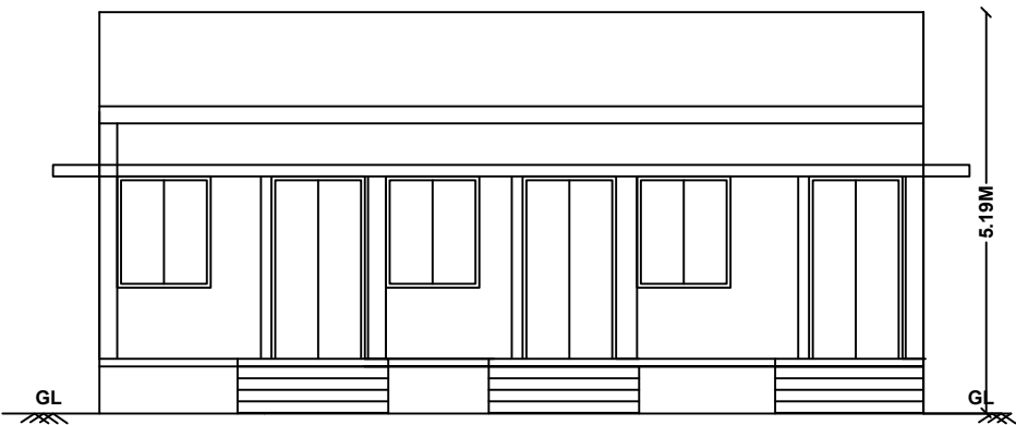
ELEVATION
