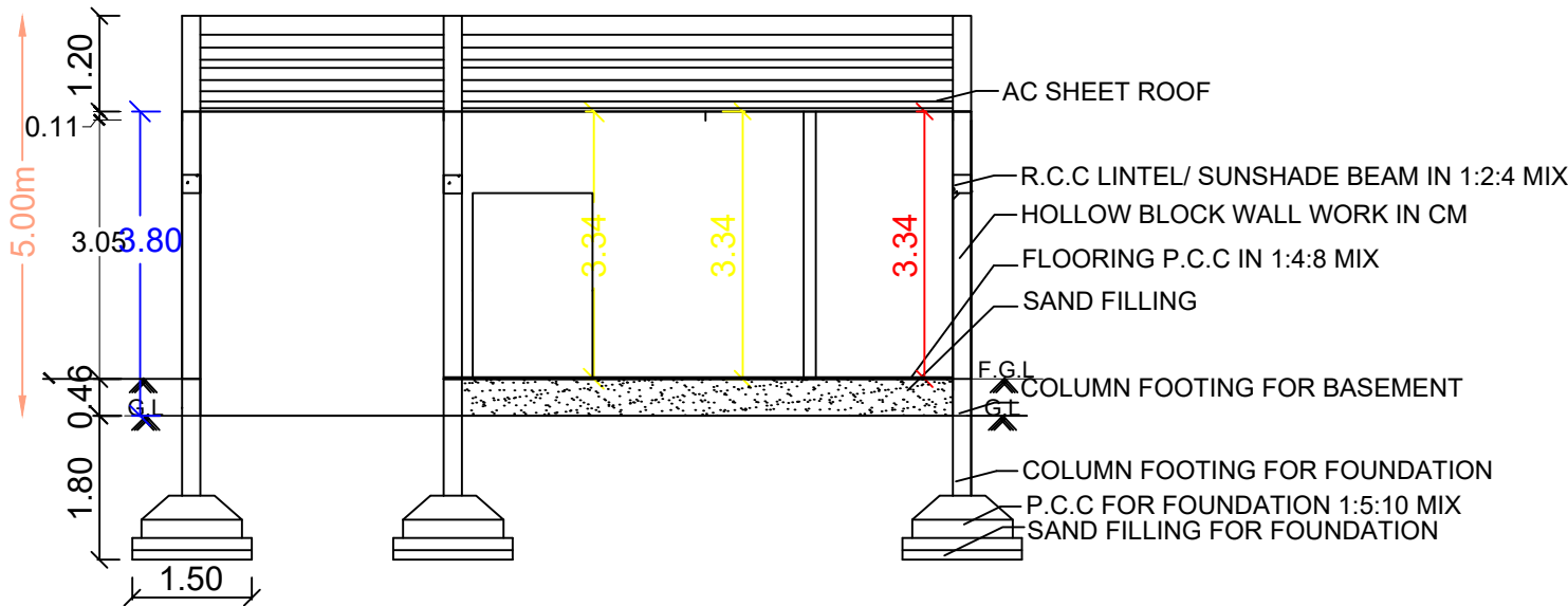
SECTION -AB
