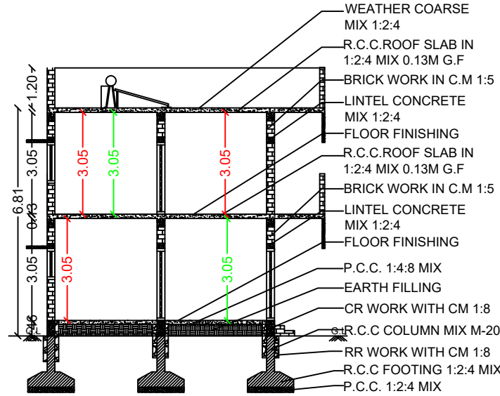
SECTION - AB
