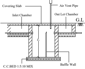
SECTION ON S.Tank [N.T.S.]
