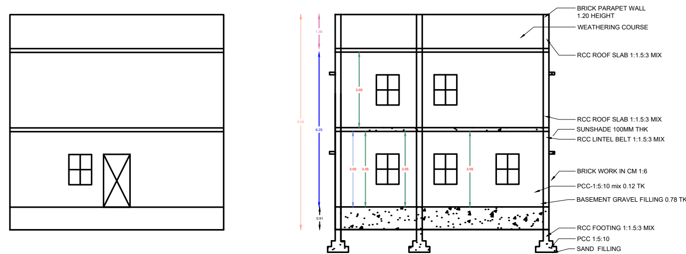
ELEVATION
