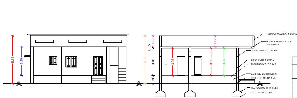
ELEVATION
