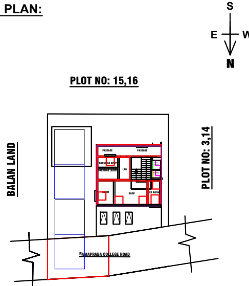
SITE PLAN:
