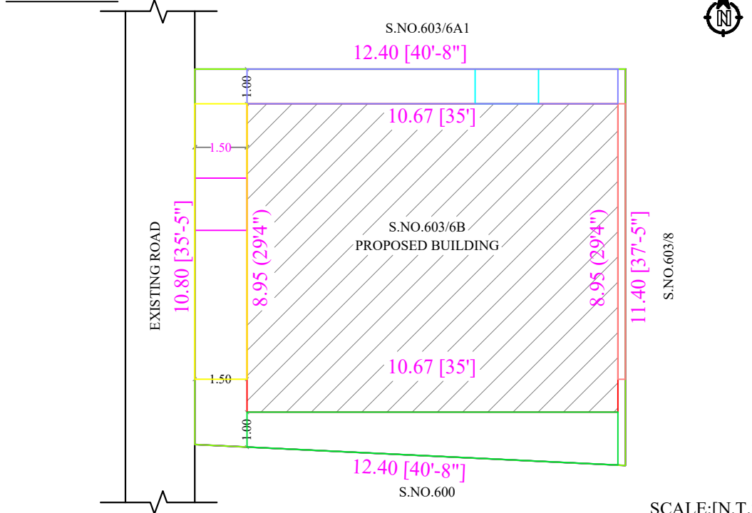
SITE PLAN :
