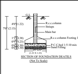
SECTION ON S.Tank [N.T.S.]
