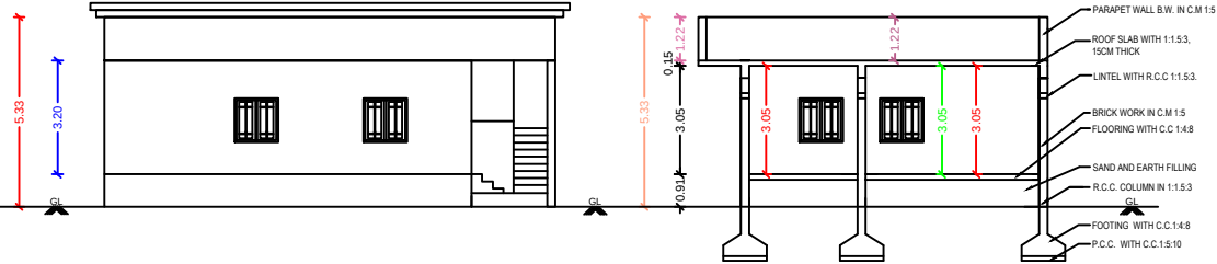
ELEVATION
