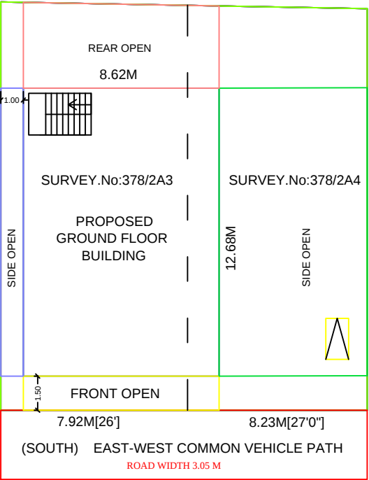
SITE PLAN(Scale 1:100)
