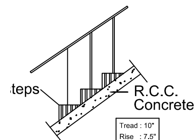
Tread : 10" Rise : 7.5"
