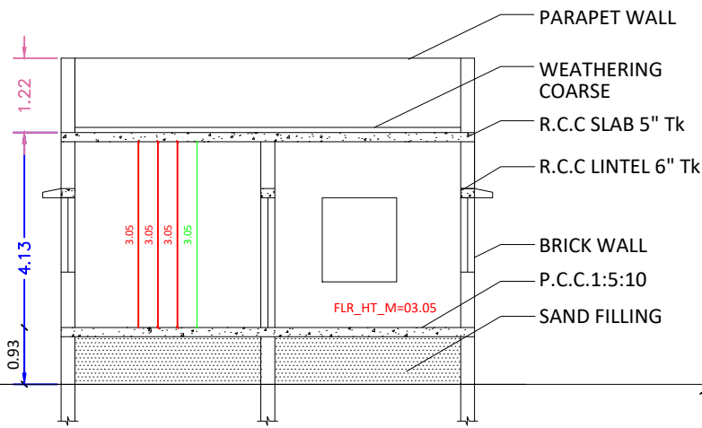
SECTION -AB
