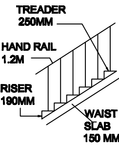
STAIR WAY-N.T.S
