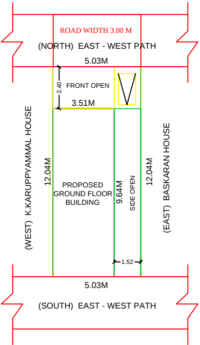
SITE PLAN(Scale 1:100)
